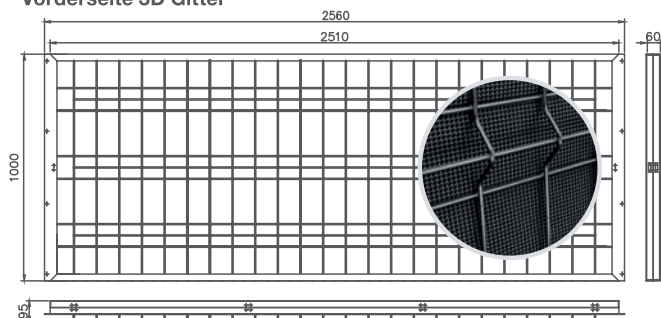
Vorderseite 3D Gitter
