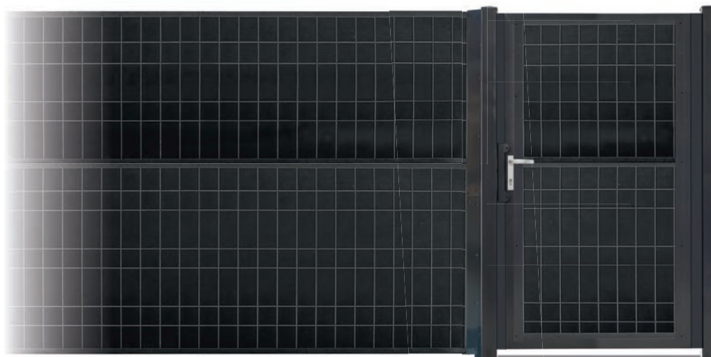
Rückseite 5/5mm Gitter
