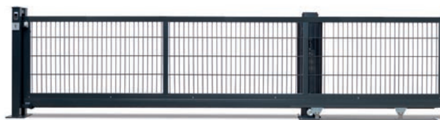
Schiebetor V-Star F60 - E-Antrieb mit Doppelstabgitter 8/6/8 mm und Antriebsäule
