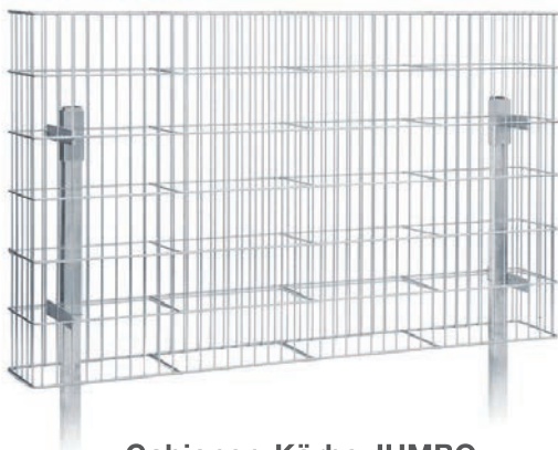
Gabionen-Körbe JUMBO Erhältliche Breiten: 1 m und 2 m Seite 134
